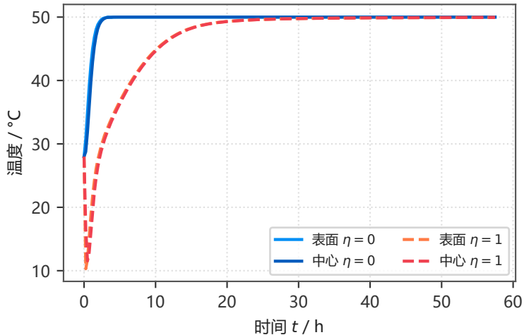
(a) 温度时程 (问题二、三, N = 400 )
