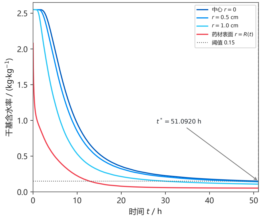
(b) 固定位置与表面含水率时程
