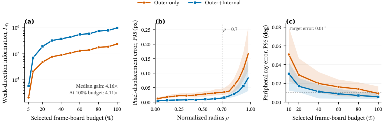
Fig. 2. 内部观测对受扰 DS 内参恢复的影响。Outer-only 与 Outer+Internal 共享相同的 Outer4 frame-board observations、受扰初值和配对噪声；Outer+Internal 仅额外加入恢复的内部格点。(a) 消除位姿后的最弱内参方向 W_1 上的 Schur 信息。(b) 在固定参考射线网格上计算的、恢复模型相对参考模型的径向像素位移 P95。(c) 不同 frame-board 预算下的外围 Ray Error P95。两种设置均从 2^\circ 外围扰动出发，并仅优化 DS 内参。图 (b) 和 (c) 汇总 100 组配对试验，曲线和阴影分别表示中位数和 IQR；外围区域定义为 \rho \geq 0.7 。
