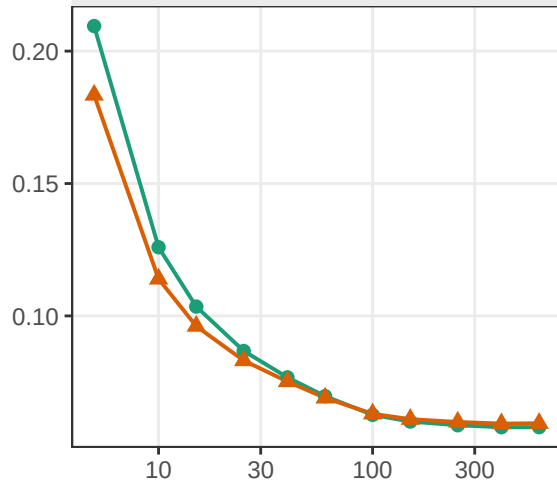
DGP 3
