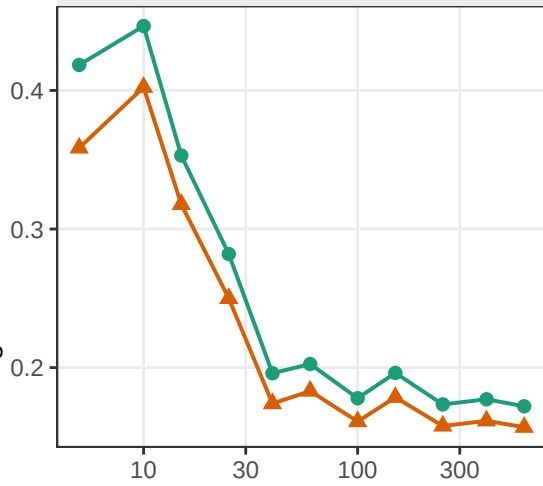
DGP 1
