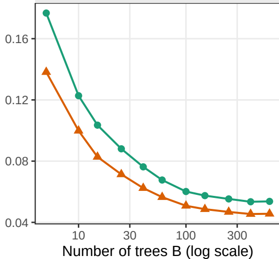
DGP 2
