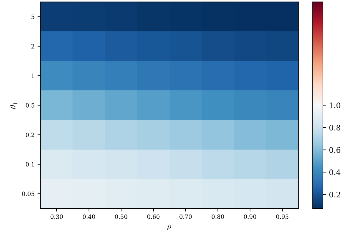
(6) E[N_1]_{C_2} / E[N_1]_A
