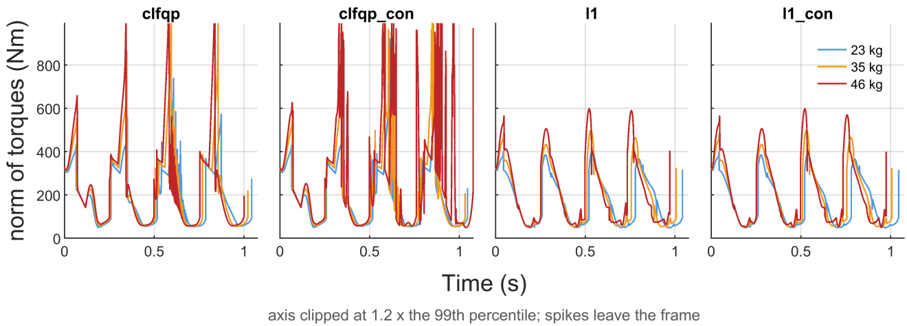
شکل ۷: بازتولید شکل 4.11. نرم گشتاورهای مفصل زیر بارهای ۲۳، ۳۵ و ۴۶ کیلوگرم روی محوری مشترک. قله گام به گام l1\_con از ۳۷۸ به ۴۷۶ و ۵۲۵ نیوتن متر می‌رسد؛ CLF-QP بدون قید در ۳۵ و ۴۶ کیلوگرم از ۱۰۰۰ نیوتن متر فراتر می‌جهد و نسخه قیددار آن اشباع می‌شود و سقوط می‌کند.
