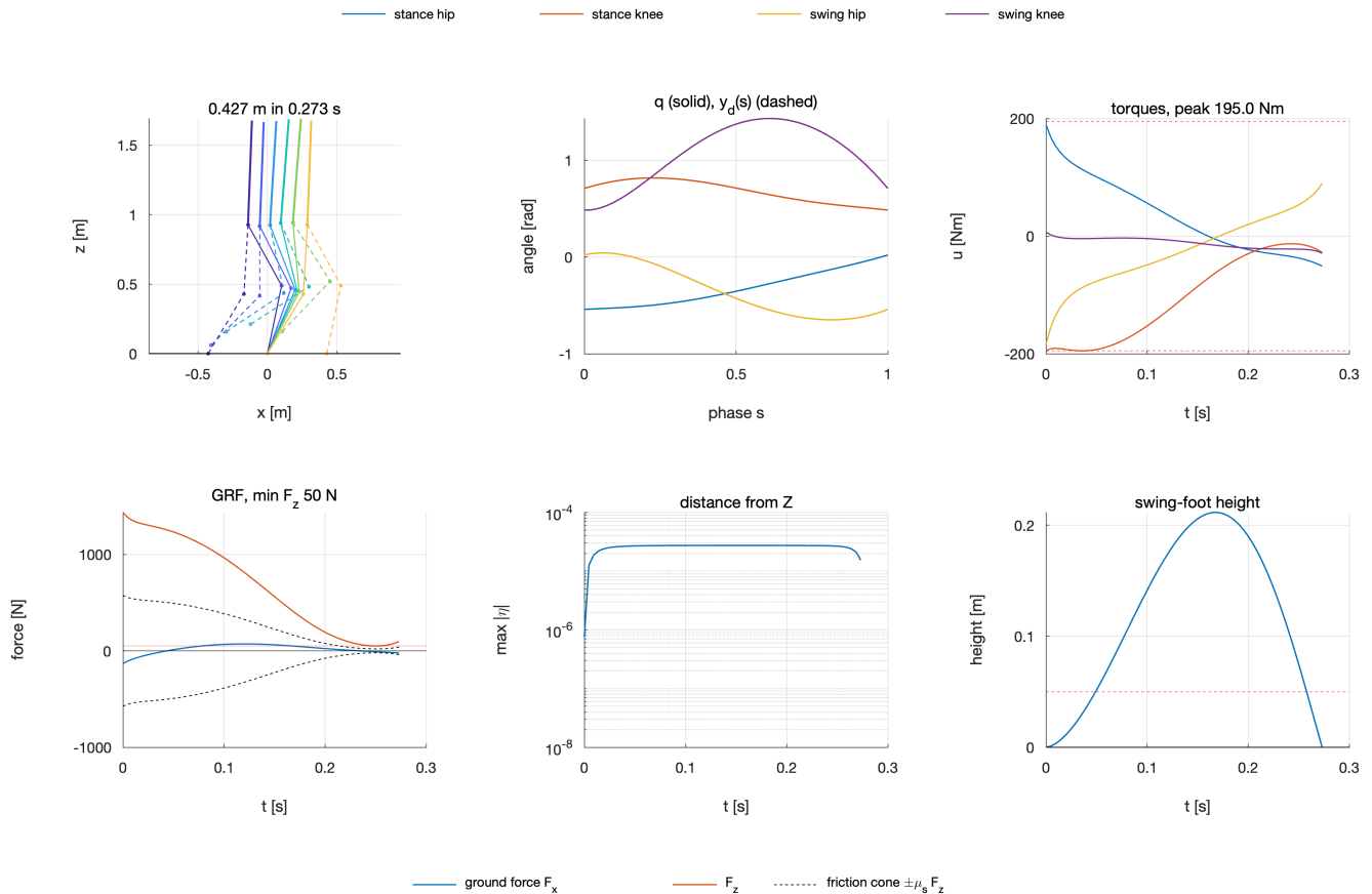
شکل ۳: گام مرجع. بالا: یک گام ۰٫۴۲۷ متری در ۰٫۲۷۳ ثانیه؛ زاویه مفاصل روی منحنی‌های بزیه؛ گشتاورها که در ابتدای گام به جعبه ۱۹۵ نیوتن‌متر می‌رسند. پایین: نیروی عمودی که درست پیش از فرود به کف ۵۰ نیوتنی می‌رسد و درون مخروط اصطکاک می‌ماند؛ فاصله از Z که تنها با پیش‌خور زیر 10^{-5} \times 3 می‌ماند؛ و ارتفاع پای نوسانی که در میانه گام از ۰٫۰۵ متر می‌گذرد و به ۰٫۲۱ متر می‌رسد.
