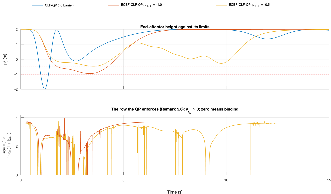
شکل ۴: ارتفاع مجری نهایی در برابر حدود مجاز. کنترل کننده مبنا در t = 1, 17 ثانیه تا 1, 98 متر سقوط می‌کند—از هر دو سطح قید عبور کرده و تقریباً به تمام دسترسی ۲- متری بازو می‌رسد. اجراهای ECBF به ترتیب در 0, 953 و 0, 464 - متوقف می‌شوند، هر کدام چند سانتی متر پیش از خط خود، و باز می‌گردند.
