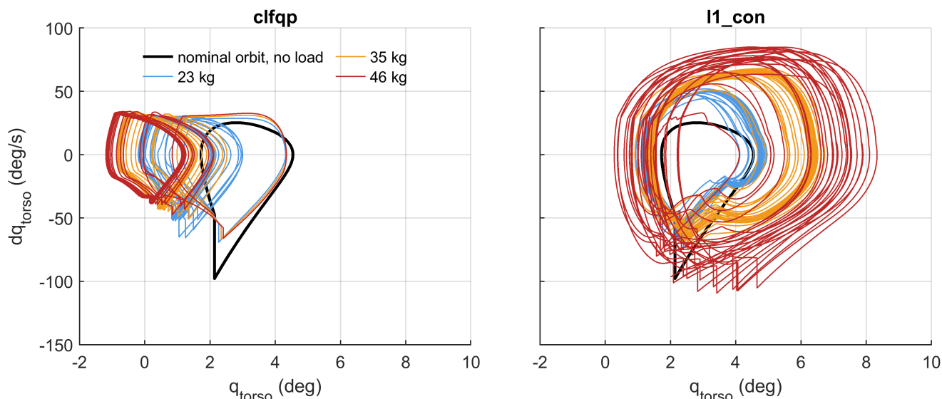
شکل ۸: تصویر فاز تنه زیر بار ثابت. مبنای بدون قید (چپ) ۲ تا ۳ درجه پایین‌تر از مدار اسمی می‌نشیند (۲، ۱- تا ۲، ۱ درجه در پنج گام آخر، در برابر ۱، ۷۲ تا ۴، ۵۵)، و چرخه l1\_con (راست) به ۰، ۶ تا ۰، ۰ درجه با نرخ گام تا ۶۸+ درجه بر ثانیه بزرگ می‌شود. بار، برخلاف مقیاس جرم، می‌تواند خود مدار را جابه‌جا کند؛ اما فاصله دو کنترل‌کننده زیر یک بار، خطای ردیابی است.
