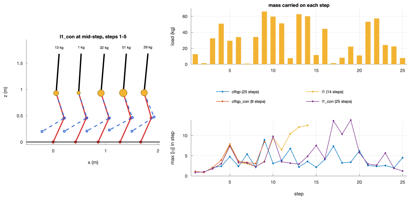
شکل ۶: بازتولید شکل 4.11 الف. سمت چپ: l1\_con در میانه گام‌های ۱ تا ۵، با اندازه دیسک ران متناسب با بار. بالا سمت راست: جرم حمل شده در هر گام. پایین سمت راست: بیشینه خطای ردیابی در هر گام. clfq\_con پس از گام ۹ و l1 پس از گام ۱۴ پایان می‌یابند؛ l1\_con هر ۲۵ گام را طی می‌کند و بزرگ‌ترین انحرافش، تا ۸، ۱۳، در گام‌های ۱۷ تا ۱۹ است.
