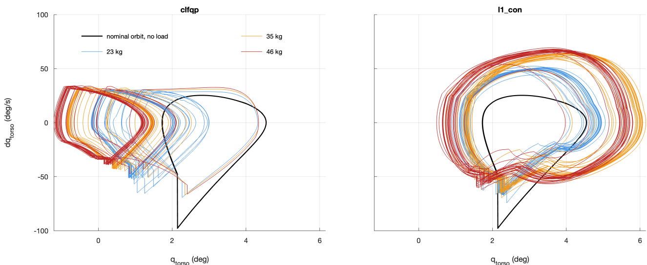
شکل ۸: تصویر فاز تنه زیر بار ثابت. مبنای بدون قید (چپ) ۲ تا ۳ درجه پایین‌تر از مدار اسمی می‌نشینند (۲، ۱- تا ۲، ۱ درجه در پنج گام آخر، در برابر ۱، ۷۲ تا ۵۵، ۴)، و چرخه l1\_con (راست) به ۰، ۶ تا ۰، ۶ درجه با نرخ گام تا ۶۸+ درجه بر ثانیه بزرگ می‌شود. بار، برخلاف مقیاس جرم، می‌تواند خود مدار را جابه‌جا کند؛ اما فاصله دو کنترل‌کننده زیر یک بار، خطای ردیابی است.
