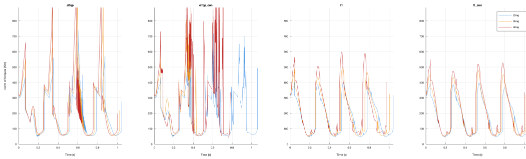
شکل ۷: بازتولید شکل 4.11. نرم گشتاورهای مفصل زیر بارهای ۲۵، ۳۵ و ۴۶ کیلوگرم روی محوری مشترک. قله گام به گام 11_con از ۳۷۸ به ۴۷۶ و ۵۲۵ نیوتن متر می‌رسد؛ CLF-QP بدون قید در ۲۵ و ۴۶ کیلوگرم از ۱۰۰۰ نیوتن متر فراتر می‌جهد و نسخه قیددار آن اشباع می‌شود و سقوط می‌کند.
