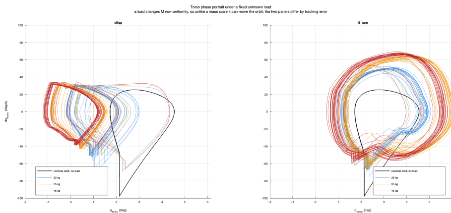
شکل ۸: تصویر فاز تنه زیر بار ثابت. مبنای بدون قید (چپ) ۲ تا ۳ درجه پایین‌تر از مدار اسمی می‌نشیند (۲، ۱- تا ۲، ۱ درجه در پنج گام آخر، در برابر ۱، ۷۲ تا ۴، ۵۵)، و چرخه 11_con (راست) به ۰، ۶ تا ۶، ۰ درجه با نرخ گام تا ۶۸+ درجه بر ثانیه بزرگ می‌شود. بار، برخلاف مقیاس جرم، می‌تواند خودِ مدار را جابه‌جا کند؛ اما فاصله دو کنترل‌کننده زیر یک بار، خطای ردیابی است.
