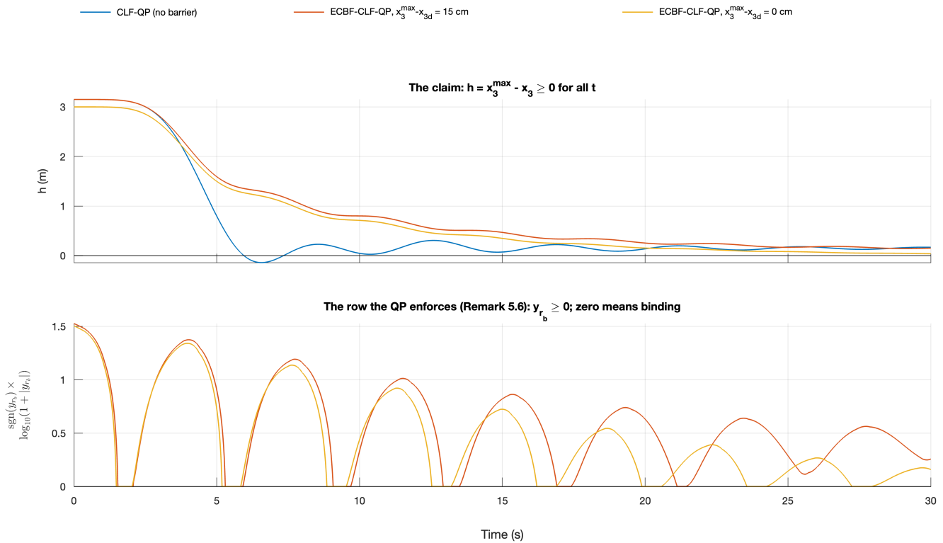
شکل ۲: بالا: مقدار تابع سد h = x_3^{\max} - x_3 در طول زمان. ادعای فصل آن است که این کمیت نامنفی بماند؛ منحنی کنترل کننده مینا این ادعا را یک بار در t = ۶, ۵۶۵ ثانیه نقض می کند. پایین: مقدار سطری که برنامه درجه دوم واقعاً اعمال می کند، روی مقیاس لگاریتمی علامت دار. مقدار صفر به معنای فعال بودن قید است؛ لمس های پیاپی همان لحظاتی هستند که سد کنترل را پس می گیرد.
