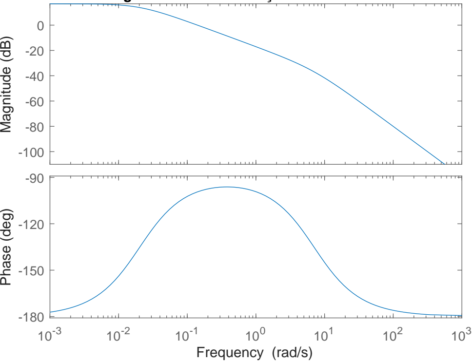
Diagrama de Bode - Função de Transferência
