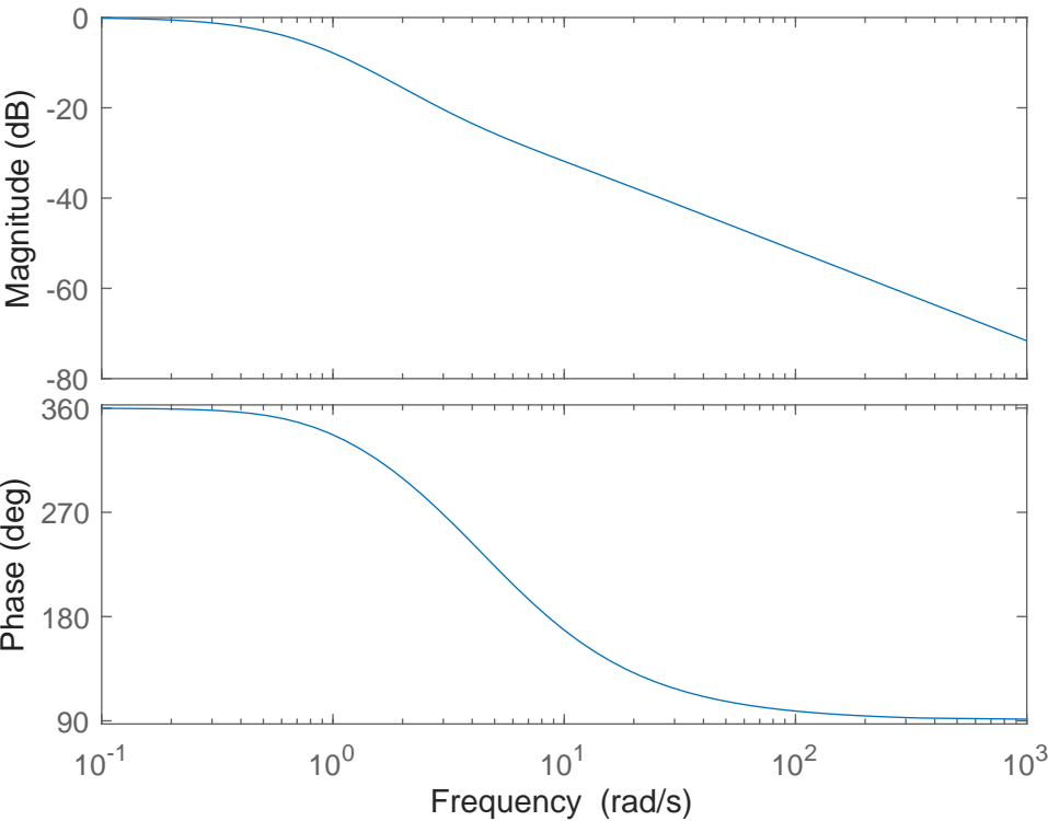
Diagrama de Bode - Sistema Controlado
