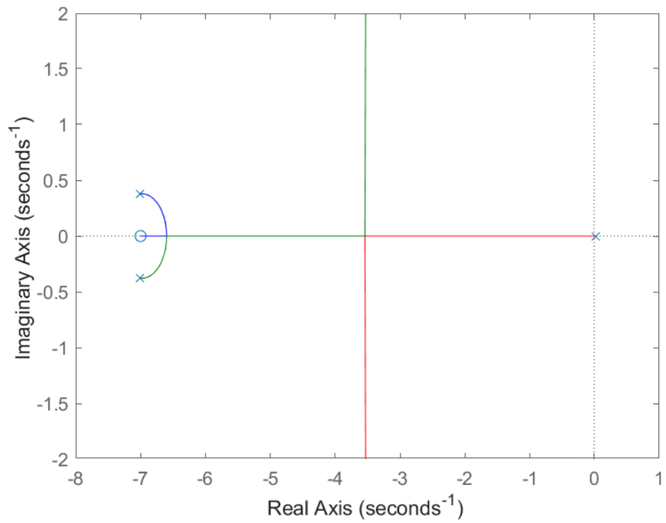
Mapa de Polos e Zeros - Função de Transferência
