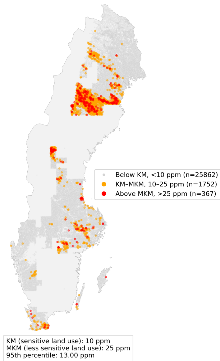
Figure 4: Arsenic vs. Naturvårdsverket guideline values (KM/MKM)
