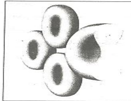
صورة مجهرية لكرات الدم الحمراء الطبيعية السليمة
