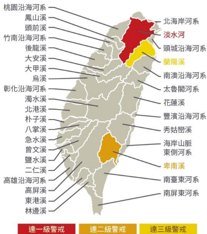
圖 36 民國 106 年 1011 豪雨應變期間各流域水位警戒圖
