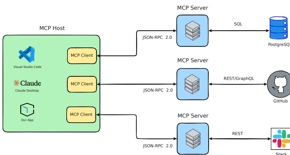
Obrázek 2.4: Ukázková architektura Client-Host-Server v rámci Model Context Protocolu.
