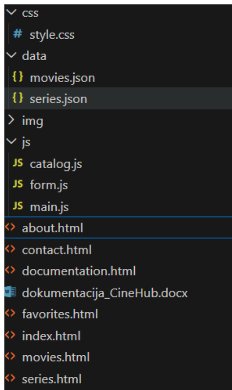
Slika 1. File tree
