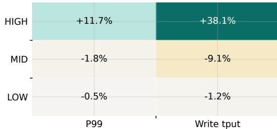
Epoch
