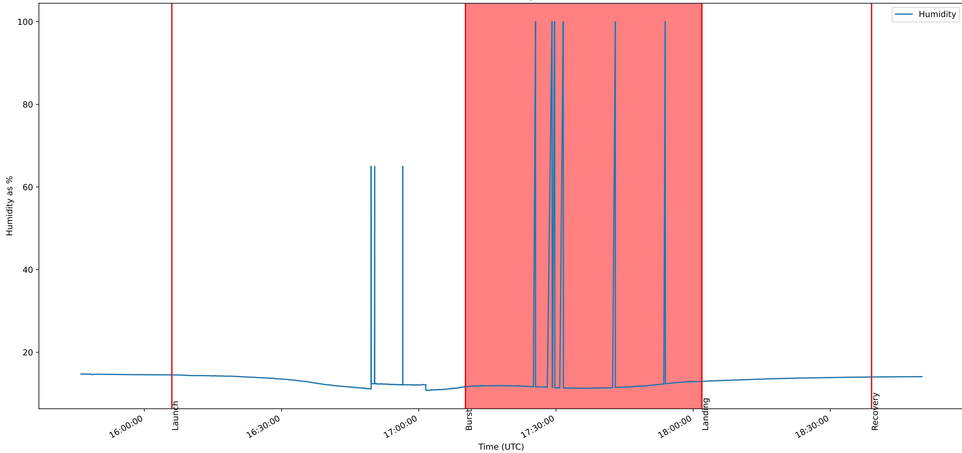
LX-179-A Humidity Plot
