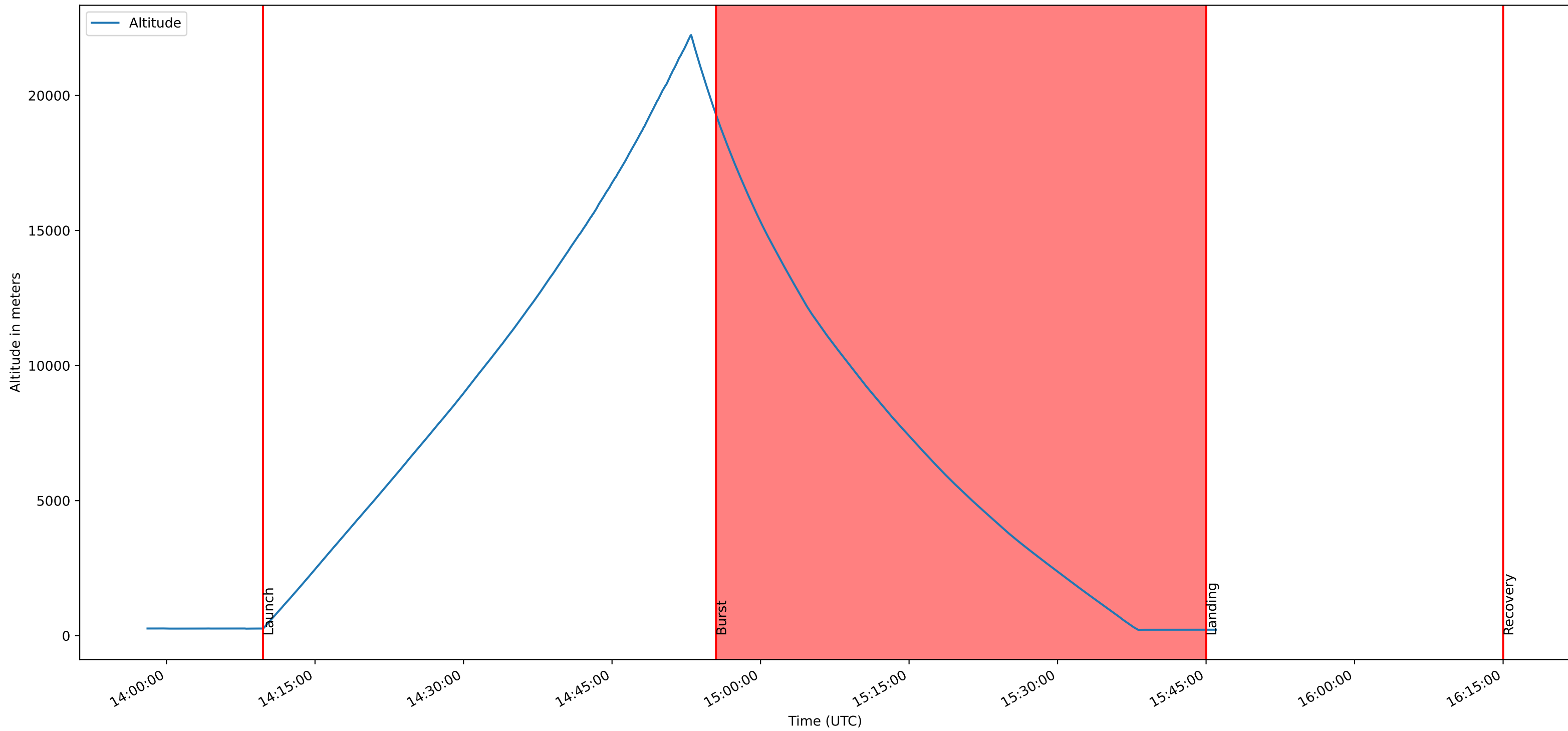
LX-187-B Altitude Plot
