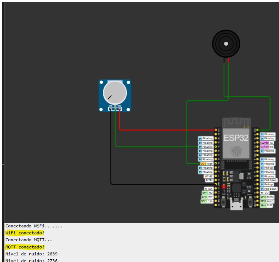
Figura 2 – Conexão do ESP32 à rede Wi-Fi e ao broker MQTT.
