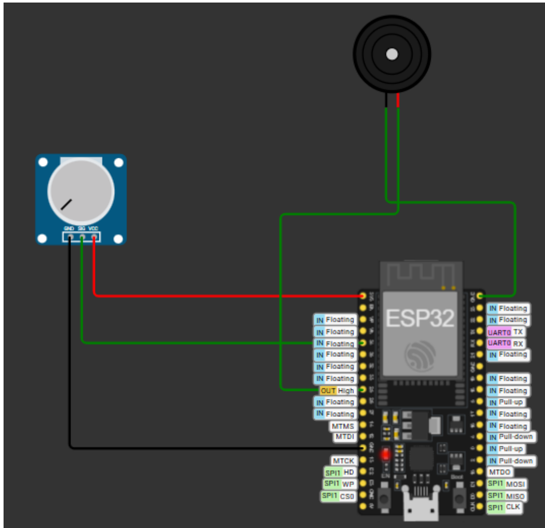
Figura 1 – Circuito eletrônico do sistema de monitoramento de ruído desenvolvido no Wokwi.
