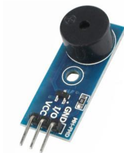
Figura 3: Buzzer (atuador sonoro)
