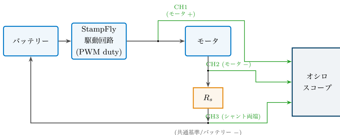
図 2 図 2：E4 シャント抵抗 + オシロスコープ 配線図。 R_s をモータ - 端子と共通基準の間に挿入し、CH1-CH2 の差動演算でモータ端子間電圧を、CH3 でシャント両端電圧（電流換算）を得る。
