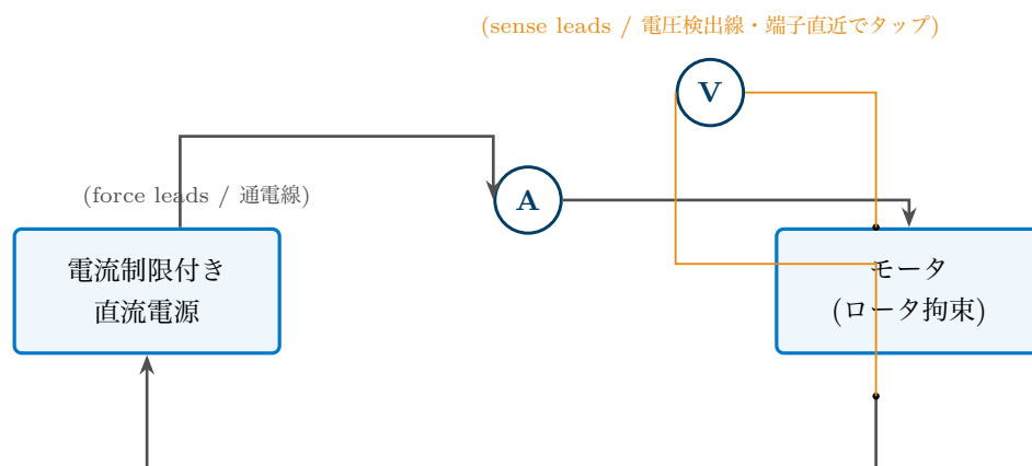
図 1 図 1：E1 4 線式 DC 測定 配線図。電流計 A は通電線に直列に挿入し、電圧計 V の検出線（オレンジ）はモータ端子直近（黒丸のタップ点）から独立に引き出す。
