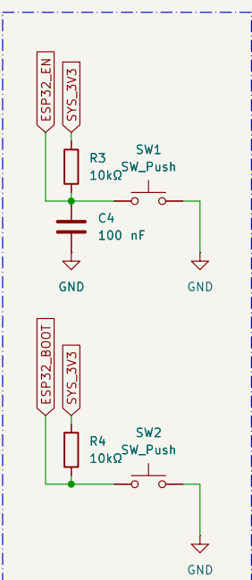
Boot & Reset
