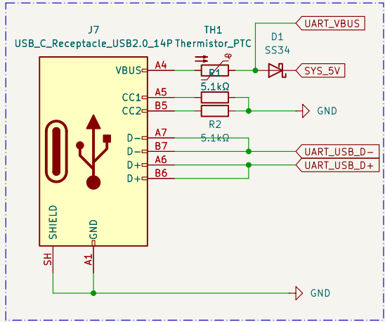
UART USB
