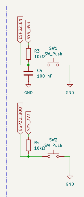
Boot & Reset
