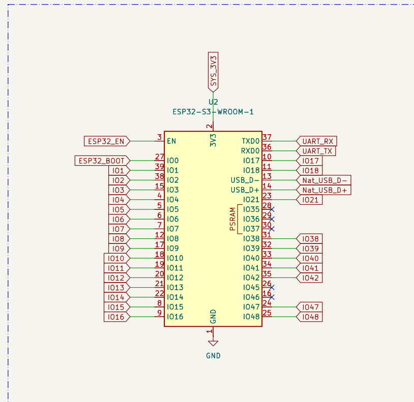
MCU
