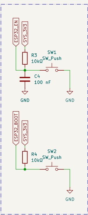
Boot & Reset
