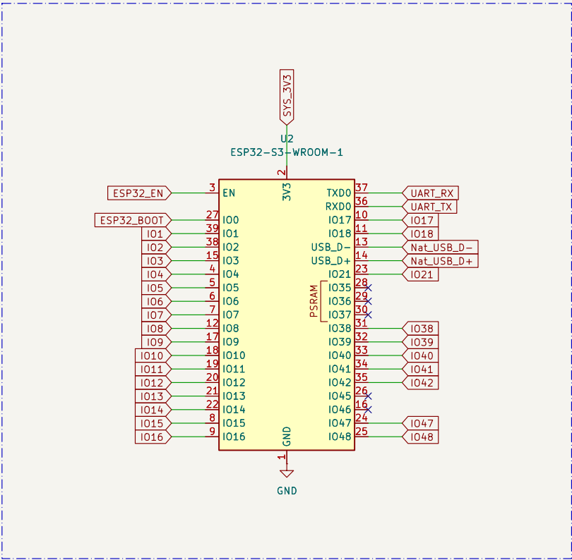
MCU
