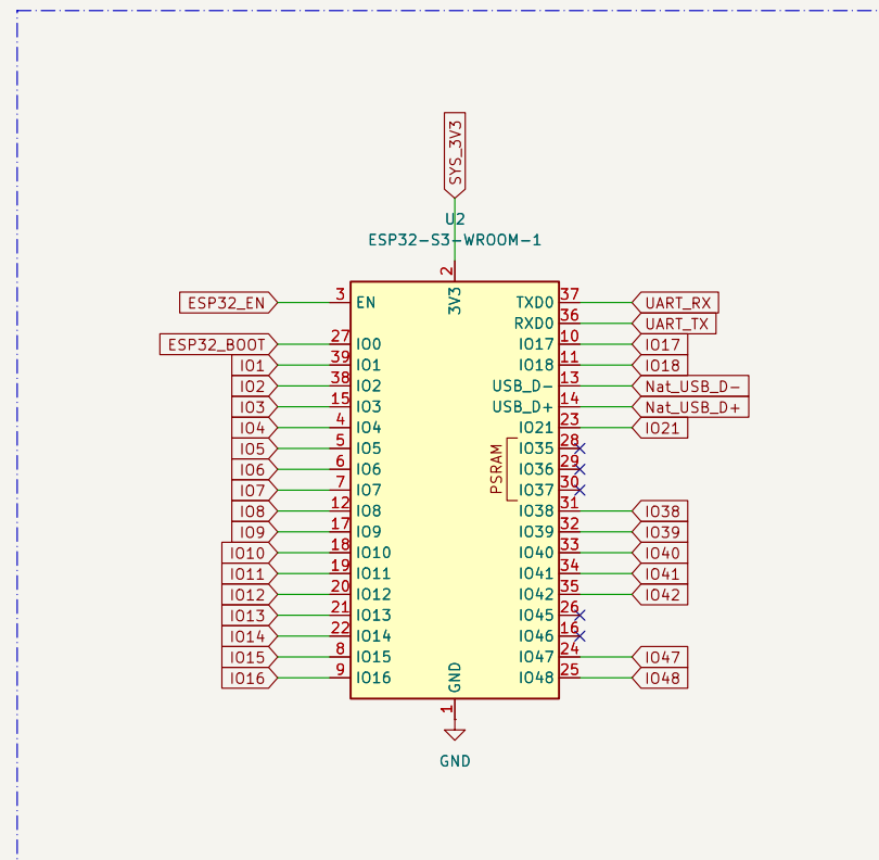
MCU
