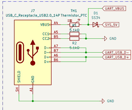
UART USB
