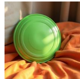
TreeGRPO
