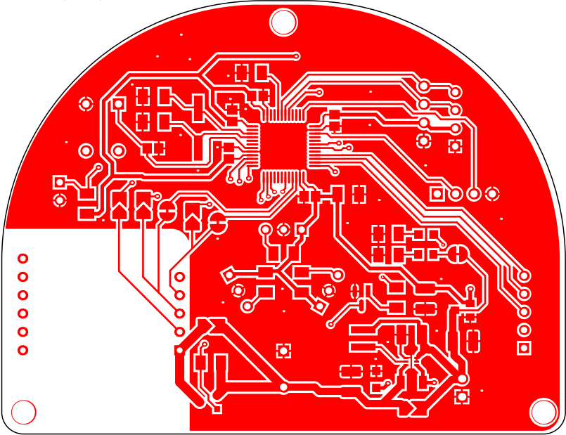
Top Layer (Scale 1.359:1)
