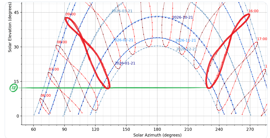
الشكل 5 رسم يوضح الاسقاط عند الساعة 9:00 صباحة على محور زاوية الظل ( \theta )
