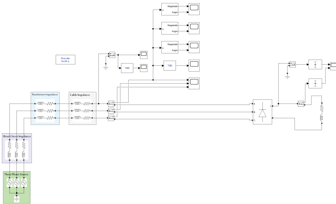
شكل 2: المخطط الكامل للدائرة بدون مرشحات
