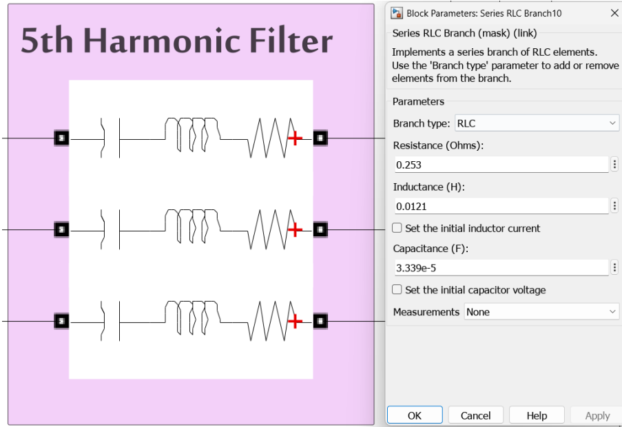
شكل 5: نافذة بارامترات مرشح التوافقية الخامسة في ماتلاب
