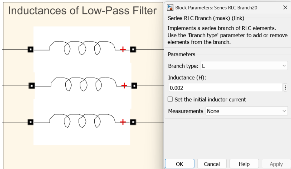
شكل 18: نافذة بارامترات ملفات الخنق في النموذج المطور
