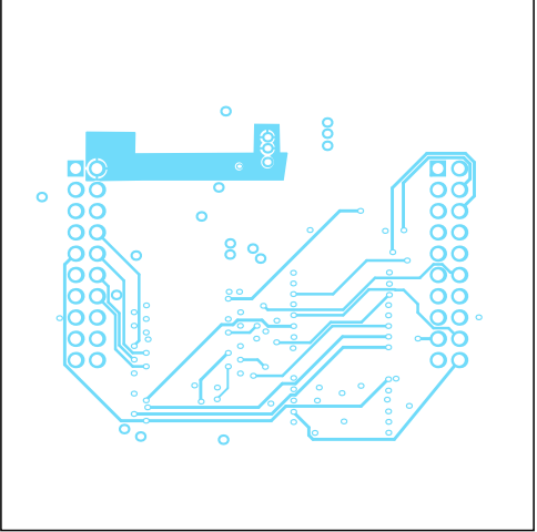
D2 (Scale 1:1)
