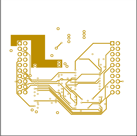
D1 (Scale 1:1)
