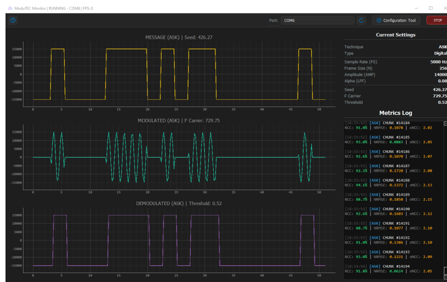
Figura 4.10: Resultados obtenidos para ASK/OOK con una secuencia digital distinta. Fuente: Elaboración propia.
