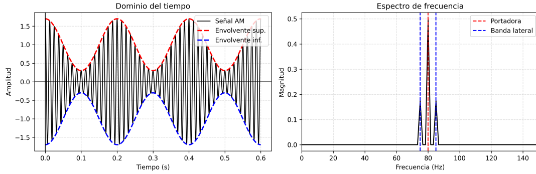
Figura 2.5: Señal modulada en amplitud (AM) en el dominio del tiempo y su representación en el dominio de la frecuencia. Fuente: Elaboración Propia.
