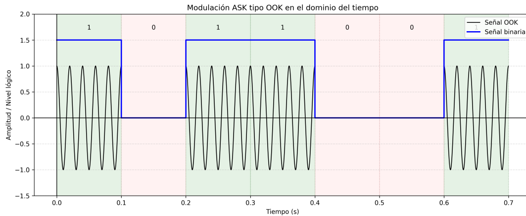
Figura 2.6: Modulación digital por amplitud tipo OOK en el dominio del tiempo. Fuente: Elaboración Propia.
