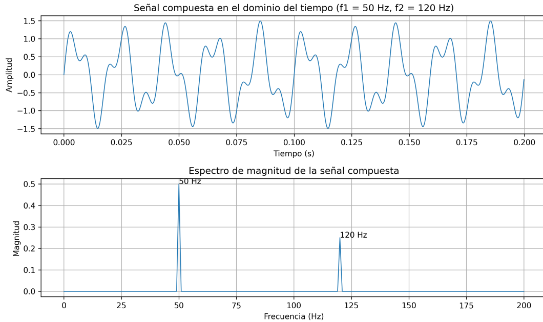
Figura 2.3: Representación de una señal compuesta en el dominio del tiempo y su correspondiente espectro de magnitud. Fuente: Elaboración Propia.
