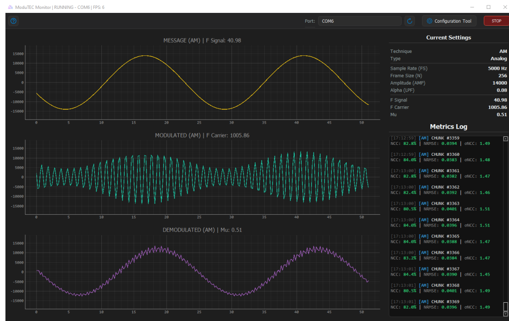
Figura 4.7: Resultados obtenidos para AM utilizando \mu = 0,51 . Fuente: Elaboración propia.
