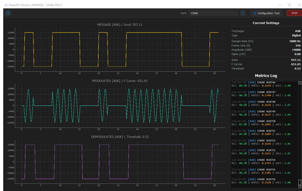
Figura 4.9: Resultados obtenidos para ASK/OOK con \tau = 0,52 . Fuente: Elaboración propia.
