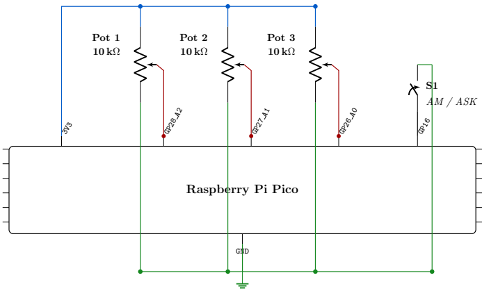
Figura 4.2: Esquemático general del módulo físico de control utilizado por el sistema embebido. Fuente: Elaboración propia.
