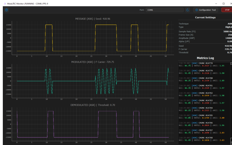
Figura 4.11: Resultados obtenidos para ASK/OOK con \tau = 0.70 . Fuente: Elaboración propia.
