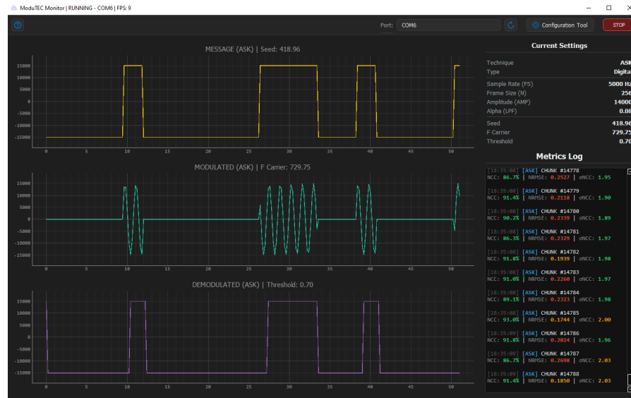
Figura 4.9: Resultados obtenidos para ASK/OOK con \tau = 0,70 . Fuente: Elaboración propia.
