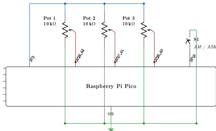
Figura 2.1: Esquemático general del m6dulo f6sico de ModuTEC.
