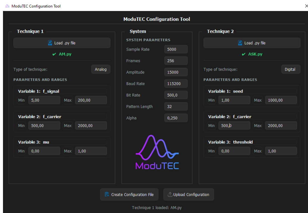
Figura B.2: Configuración personalizada ingresada en Config Tool.
