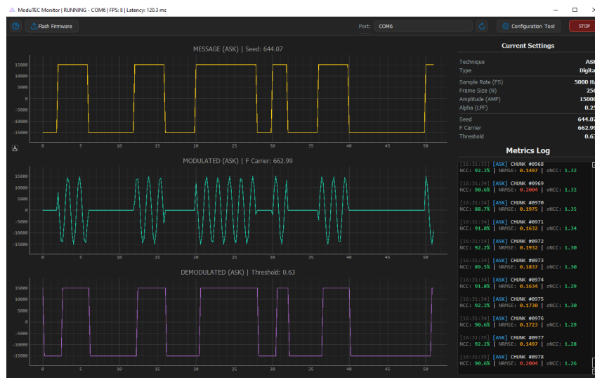
Figura B.5: Cambio de técnica activa mediante el interruptor físico del módulo.
