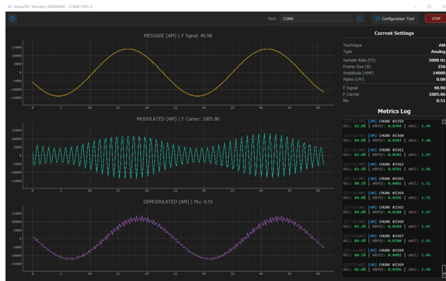
Figura 4.6: Resultados obtenidos para AM utilizando \mu = 0,51 . Fuente: Elaboración propia.
