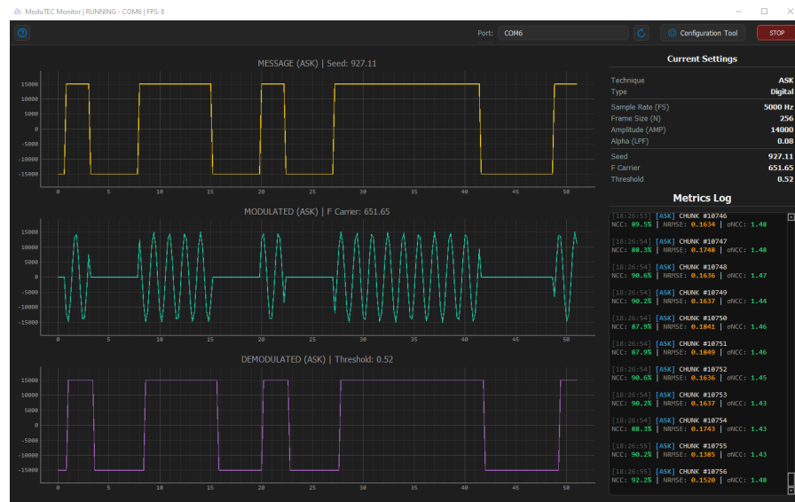
Figura 4.8: Resultados obtenidos para ASK/OOK con \tau = 0,52 . Fuente: Elaboración propia.
