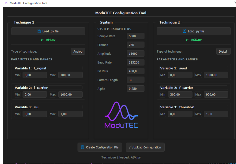
Figura 4.11: Herramienta de configuración desarrollada para la parametrización dinámica del sistema. Fuente: Elaboración propia.
