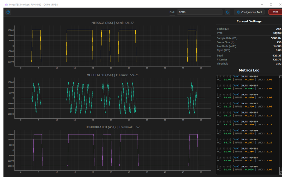
Figura 4.9: Resultados obtenidos para ASK/OOK con una secuencia digital distinta. Fuente: Elaboración propia.
