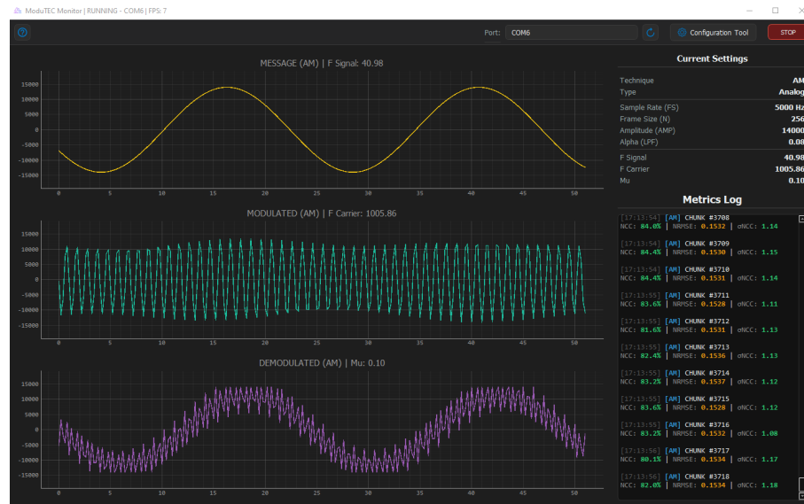
Figura 4.6: Resultados obtenidos para AM utilizando \mu = 0,10 . Fuente: Elaboración propia.
