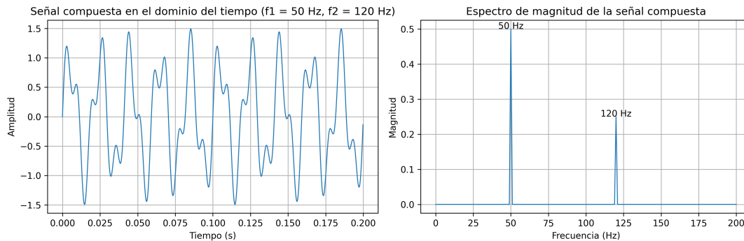
Figura 2.3: Representación de una señal compuesta en el dominio del tiempo y su correspondiente espectro de magnitud. Fuente: Elaboración Propia.
