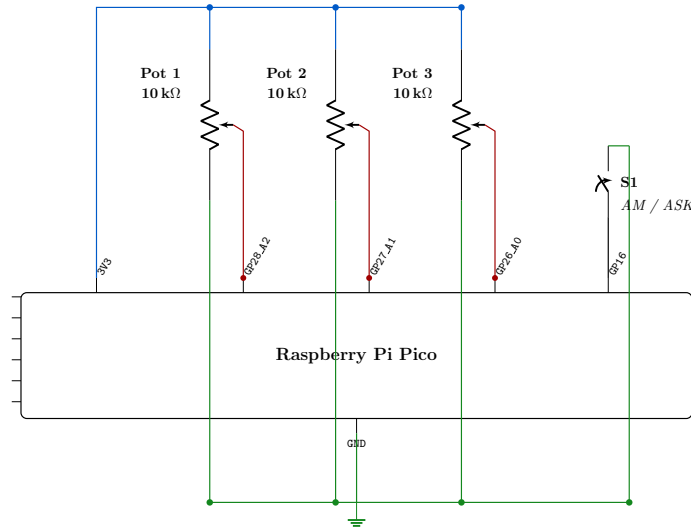
Figura 4.2: Esquemático general del módulo físico de control utilizado por el sistema embebido. Fuente: Elaboración propia.
