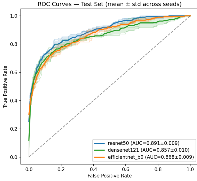
Fig. 2. ROC eğrisi karşılaştırması (tüm tohumlar). ResNet-50 en yüksek ortalama AUC'yi verir.
