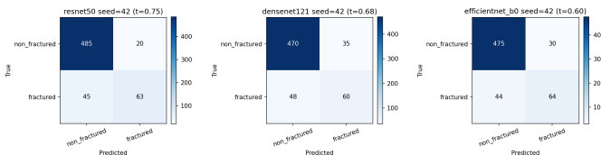
Fig. 4. Karışıklık matrisleri (tohum 42): soldan sağa ResNet-50, DenseNet-121, EfficientNet-B0. Hataların çoğu yanlış negatif (kaçırılan kırık) yönündedir.
