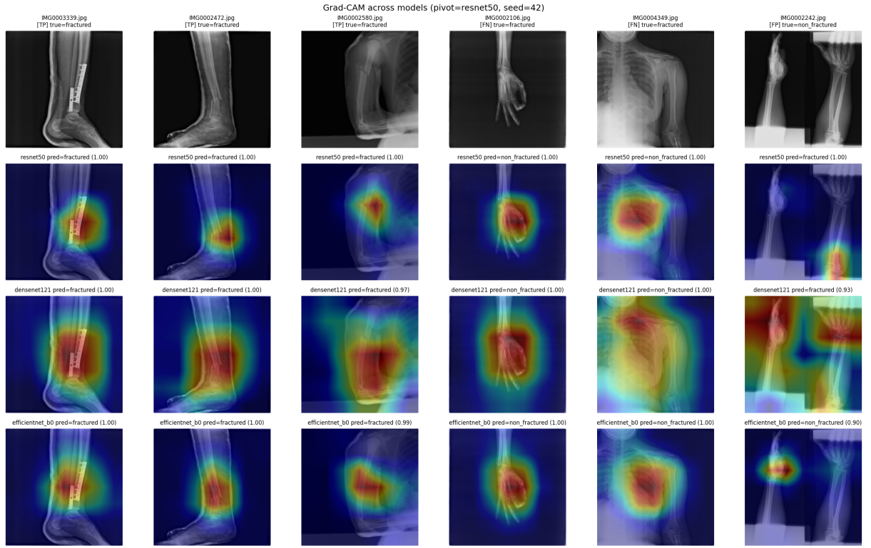
Fig. 5. Grad-CAM ısı haritaları (tohum 42). Doğru kararlarda etkinleşme kırık bölgesinde toplanır; hatalı örneklerde dağılır.
