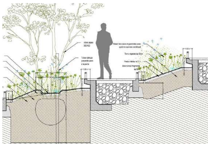
Coupe des emmarchements et détail de plantation
