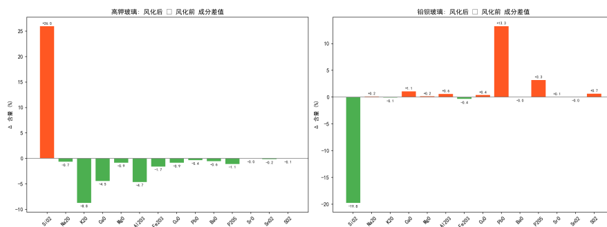
图 4: 风化效应差值棒图（高钾 vs 铅钡）
