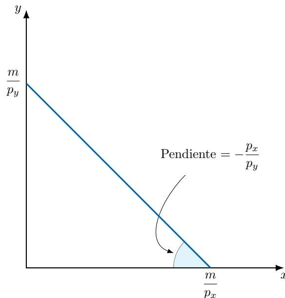
Figura 3.4: Restricción presupuestaria
