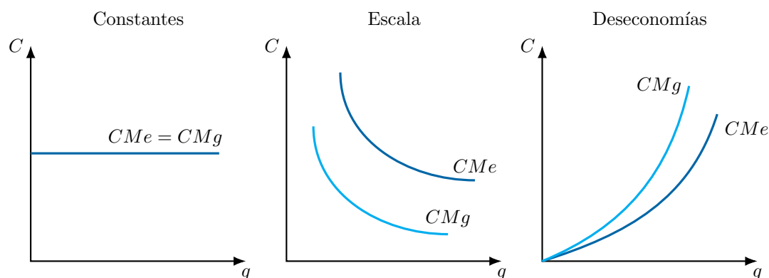
Figura 6.6: Curvas de coste sin rendimientos mixtos
