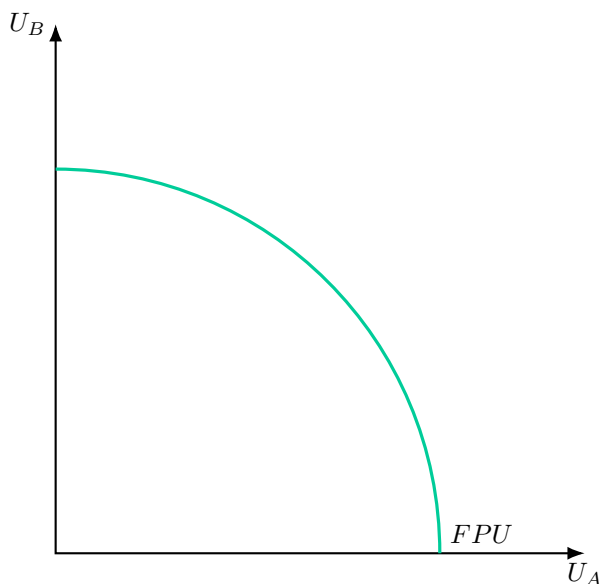
Figura 14.4: Frontera de posibilidades de utilidad
