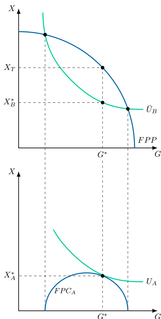
Figura 15.2: Condición de Samuelson
