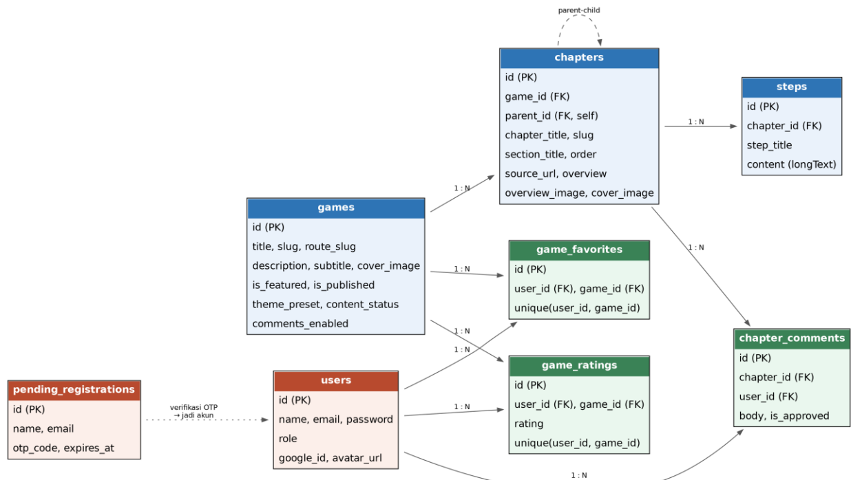
Gambar: Entity Relationship Diagram (ERD) ringkas seluruh tabel pada Walkthrough Game Hub.
