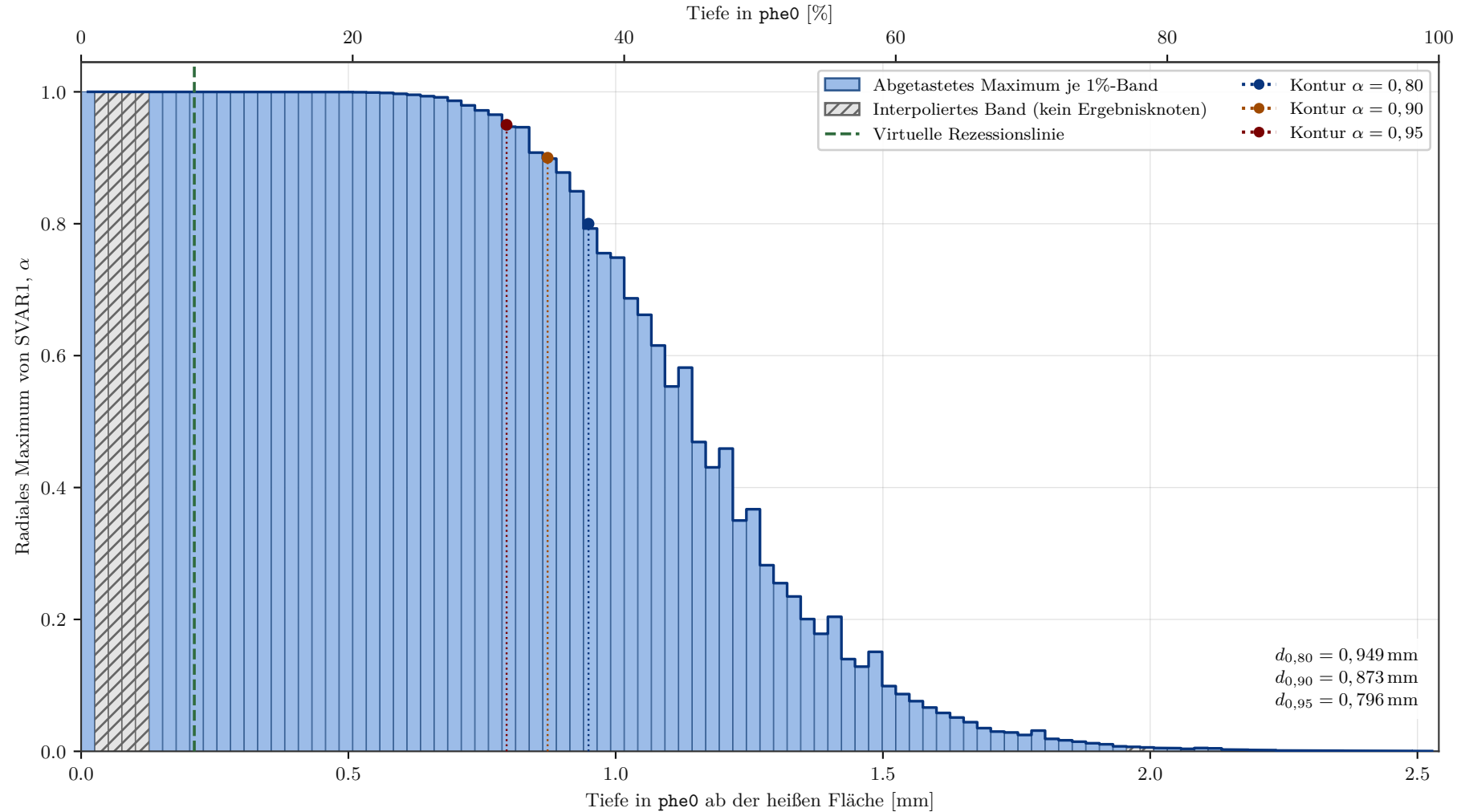
Simulation 2: radiales SVAR1-Profil im letzten extrahierten Zustand t = 6,4500\text{ s} ; Rezessionslinie s = 0,212\text{ mm}
