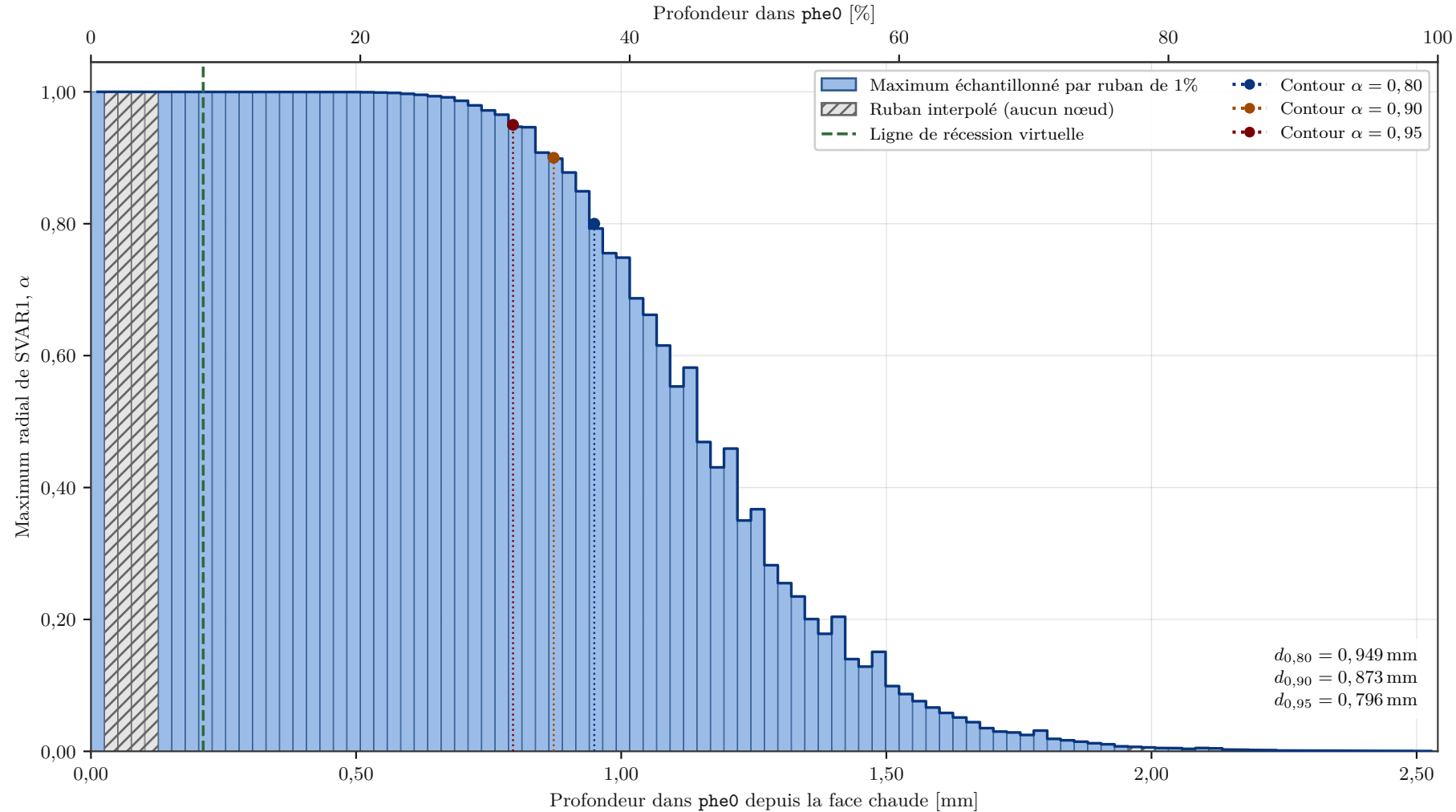
Simulation 2 : profil radial de SVAR1 au dernier état extrait t = 6,4500 \text{ s} ; ligne de récession s = 0,212 \text{ mm}
