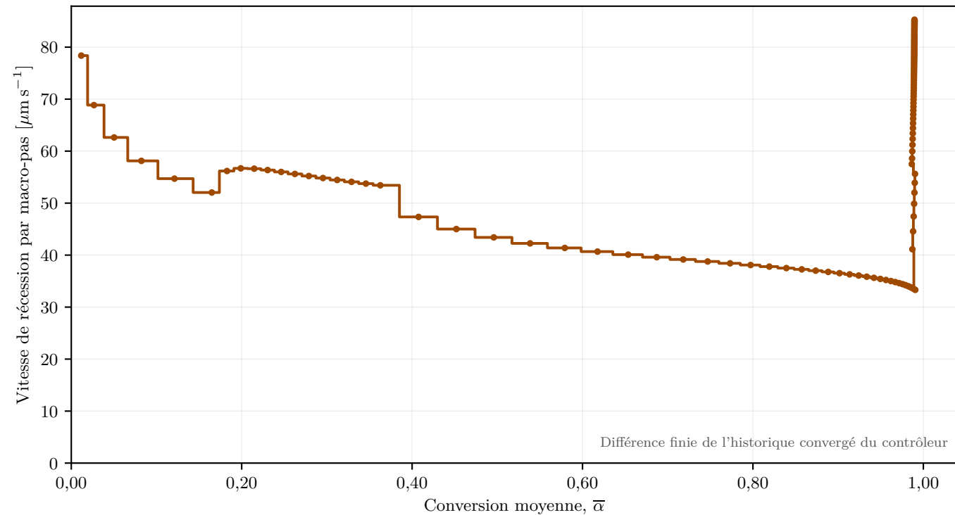
Vitesse de récession en fonction de la conversion moyenne
