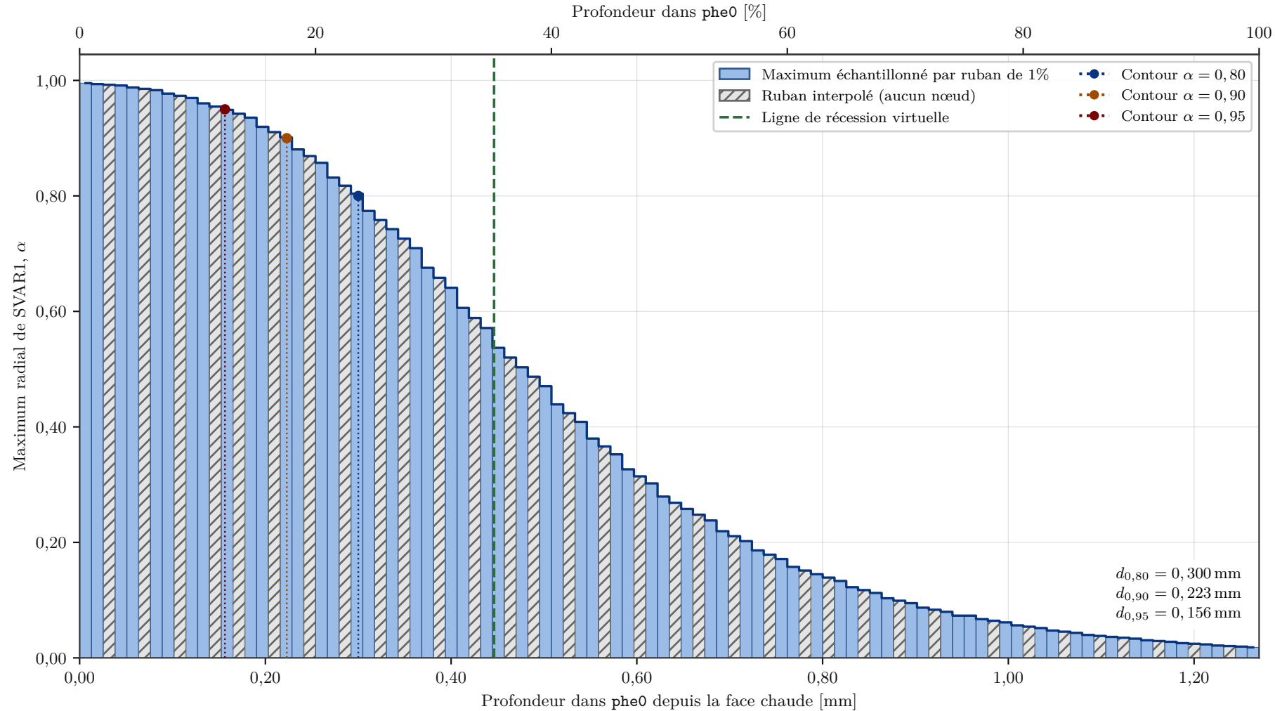
Simulation 3 : profil radial de SVAR1 au dernier état extrait t = 7,0000 \text{ s} ; ligne de récession s = 0,446 \text{ mm}
