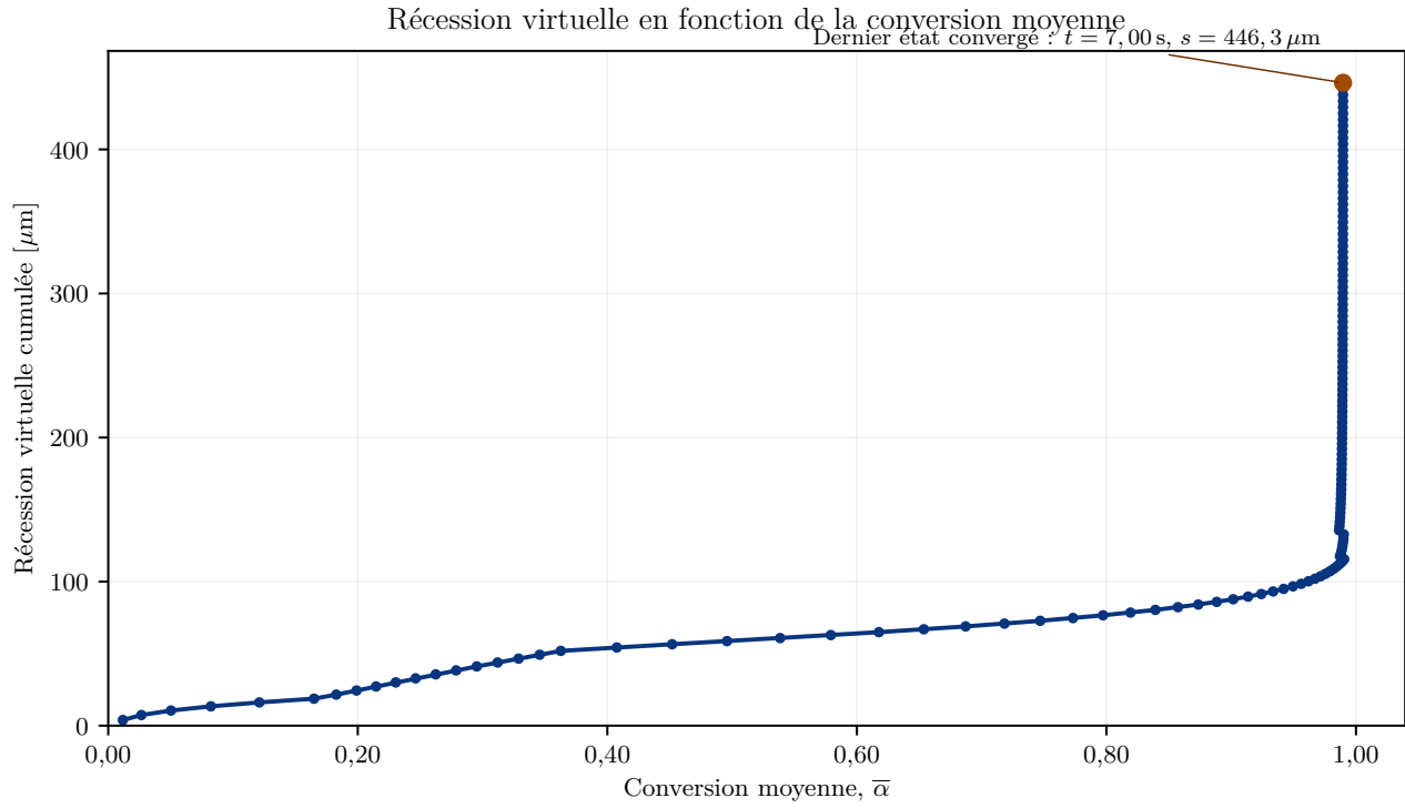
Figure 23. Récession virtuelle cumulée en fonction de la conversion moyenne de la couche active.
