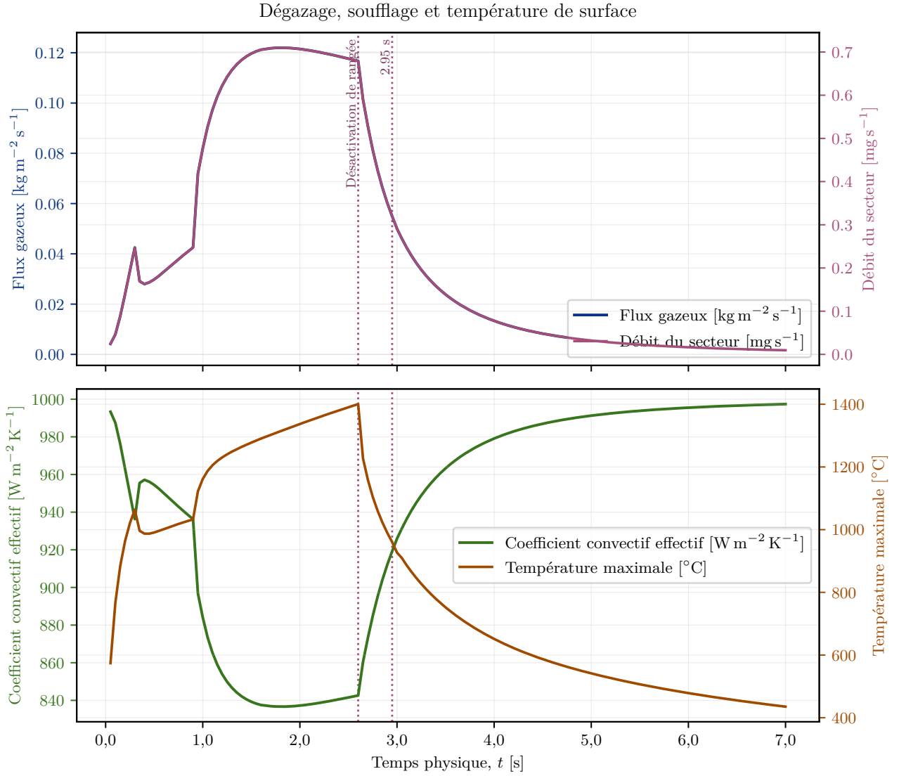
Figure 20. Évolution du dégazage, du coefficient convectif effectif et de la température maximale de la surface chaude. Le débit total représenté est celui du secteur de 0,10^{\circ} .
