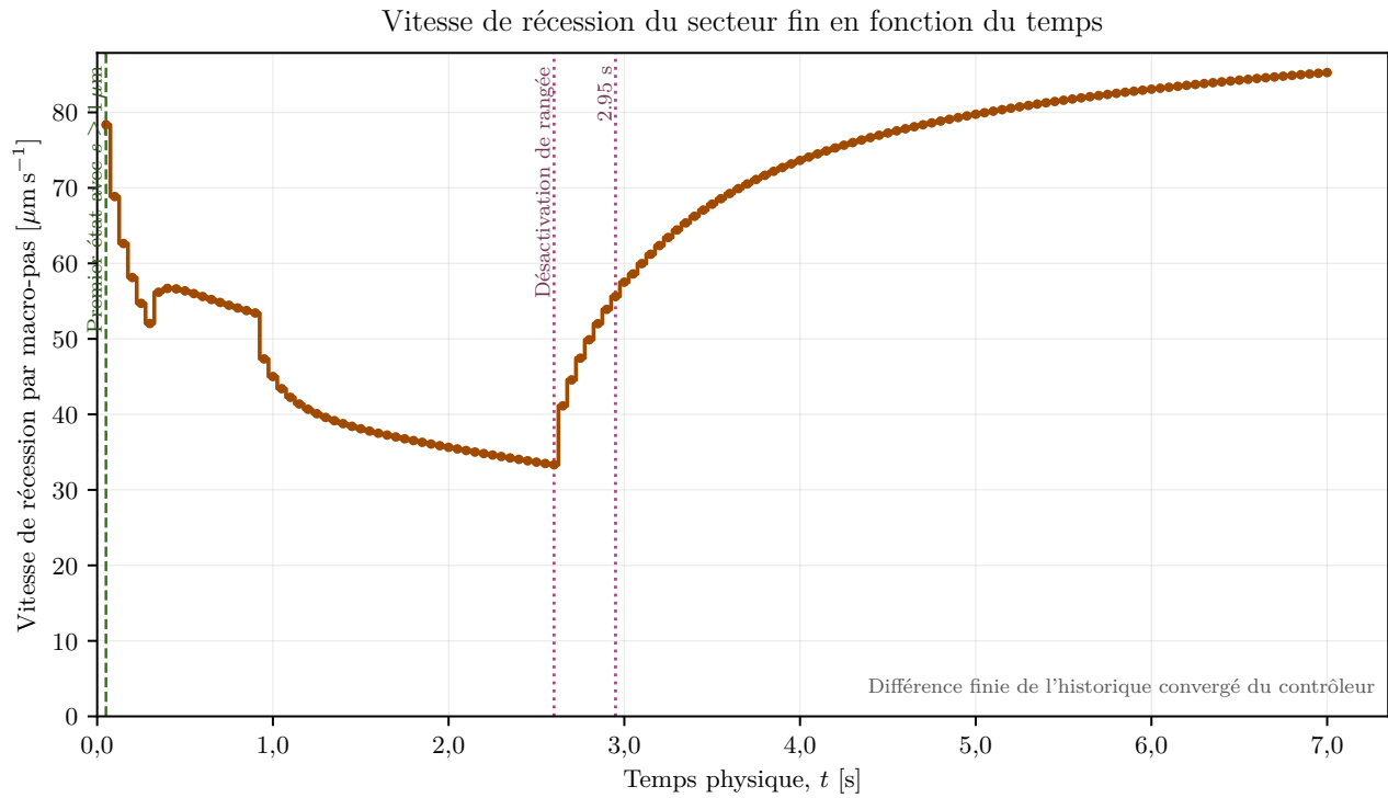
Figure 22. Vitesse moyenne de récession par macro-pas. Il s'agit d'une dérivée temporelle de l'historique du contrôleur, sans barre d'écart-type spatial.
