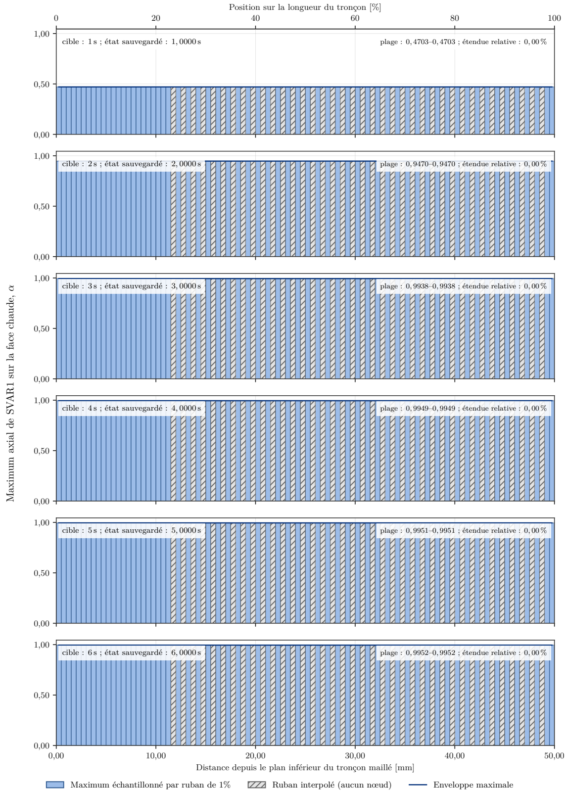
Figure 28. Uniformité axiale de SVAR1 sur la face chaude du secteur fin.
