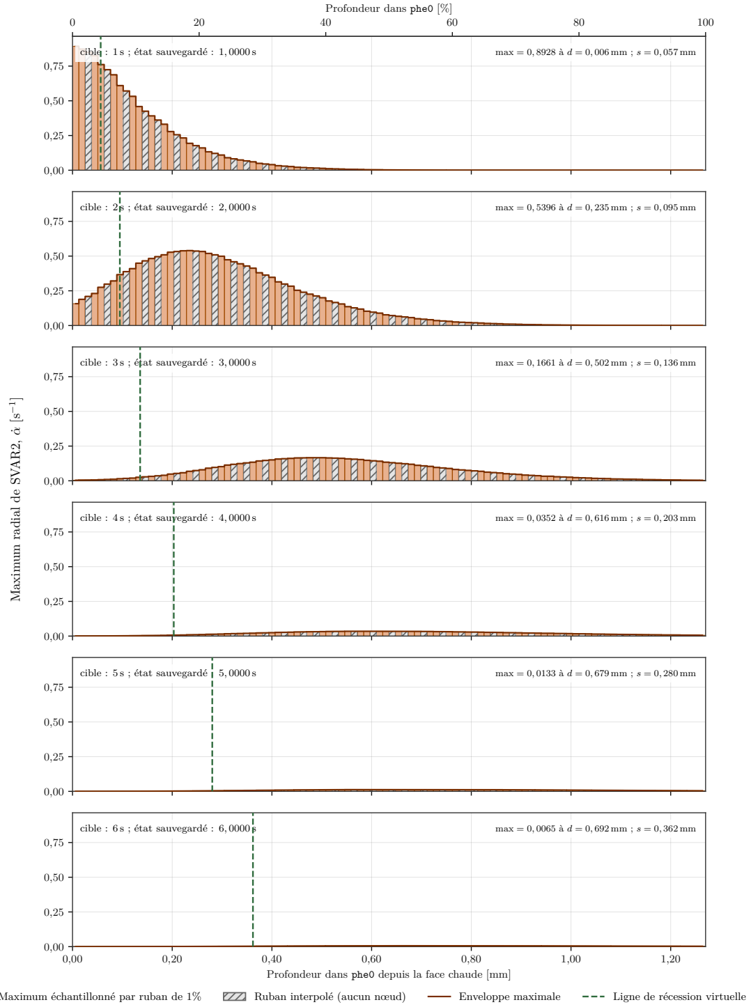
Figure 27. Évolution des profils radiaux de SVAR2 ; le maximum localise la zone de pyrolyse encore active.
