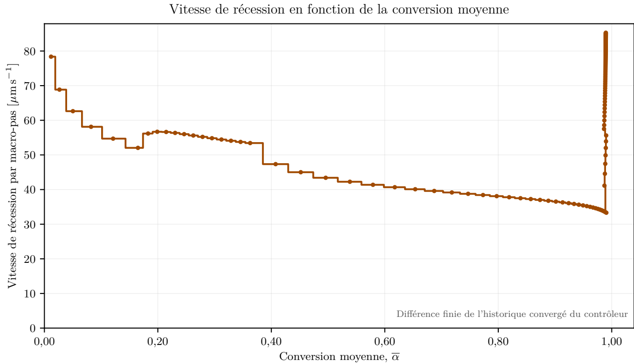
Figure 24. Vitesse de récession par macro-pas en fonction de la conversion moyenne.
