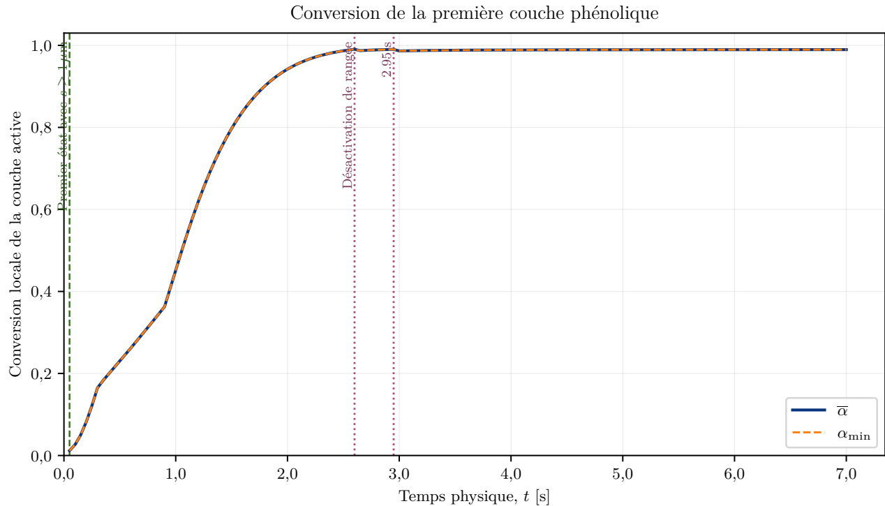
Figure 19. Conversion moyenne et minimale enregistrées dans la couche active du secteur fin sur les 140 états convergés. Les lignes verticales marquent les deux désactivations de rangées.
