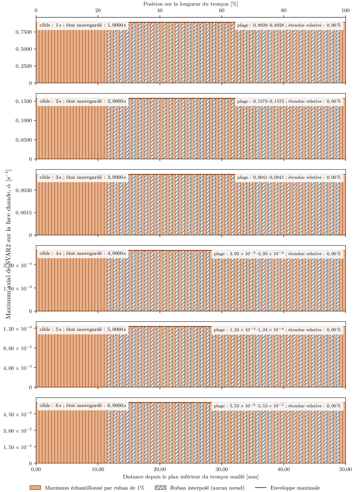
Figure 29. Uniformité axiale de SVAR2 sur la face chaude du secteur fin.
