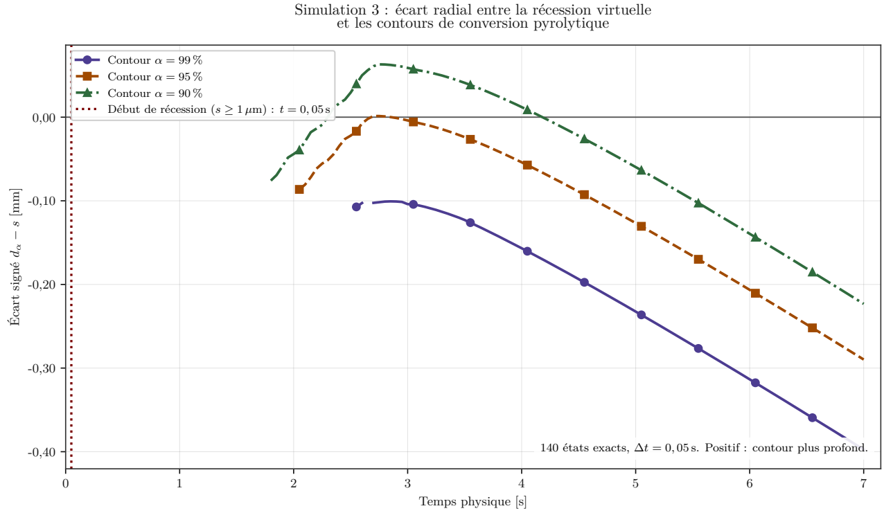
Figure 30. Écart signé entre la ligne de récession et les contours de conversion à 99 %, 95 % et 90 % sur les 140 états. Une valeur positive place le contour plus profondément dans la paroi. La ligne verticale marque la première récession numériquement significative.
