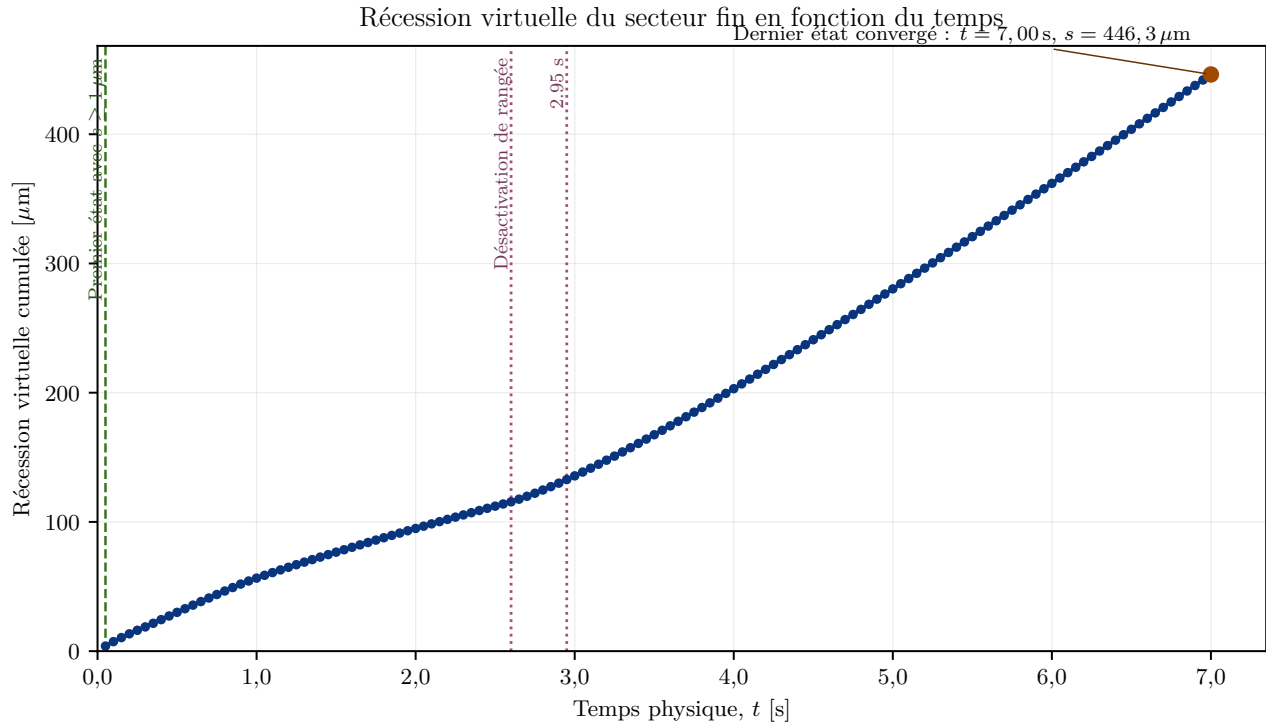
Figure 21. Récession virtuelle cumulée en fonction du temps pour la simulation 3. Les lignes verticales repèrent l'apparition numérique du front de récession et les deux désactivations de rangées.
