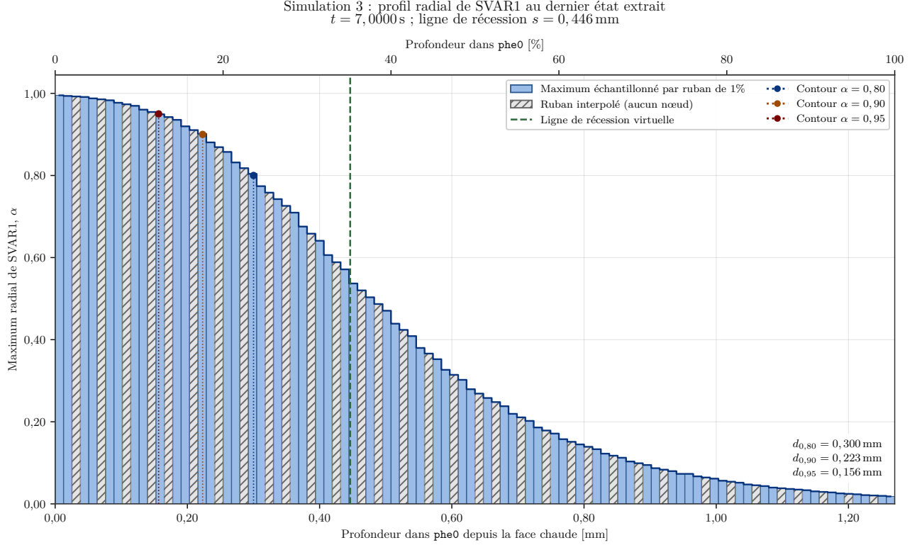
Figure 25. Profil radial final de SVAR1 à 7 s, avec les contours de conversion et la ligne de récession virtuelle.
