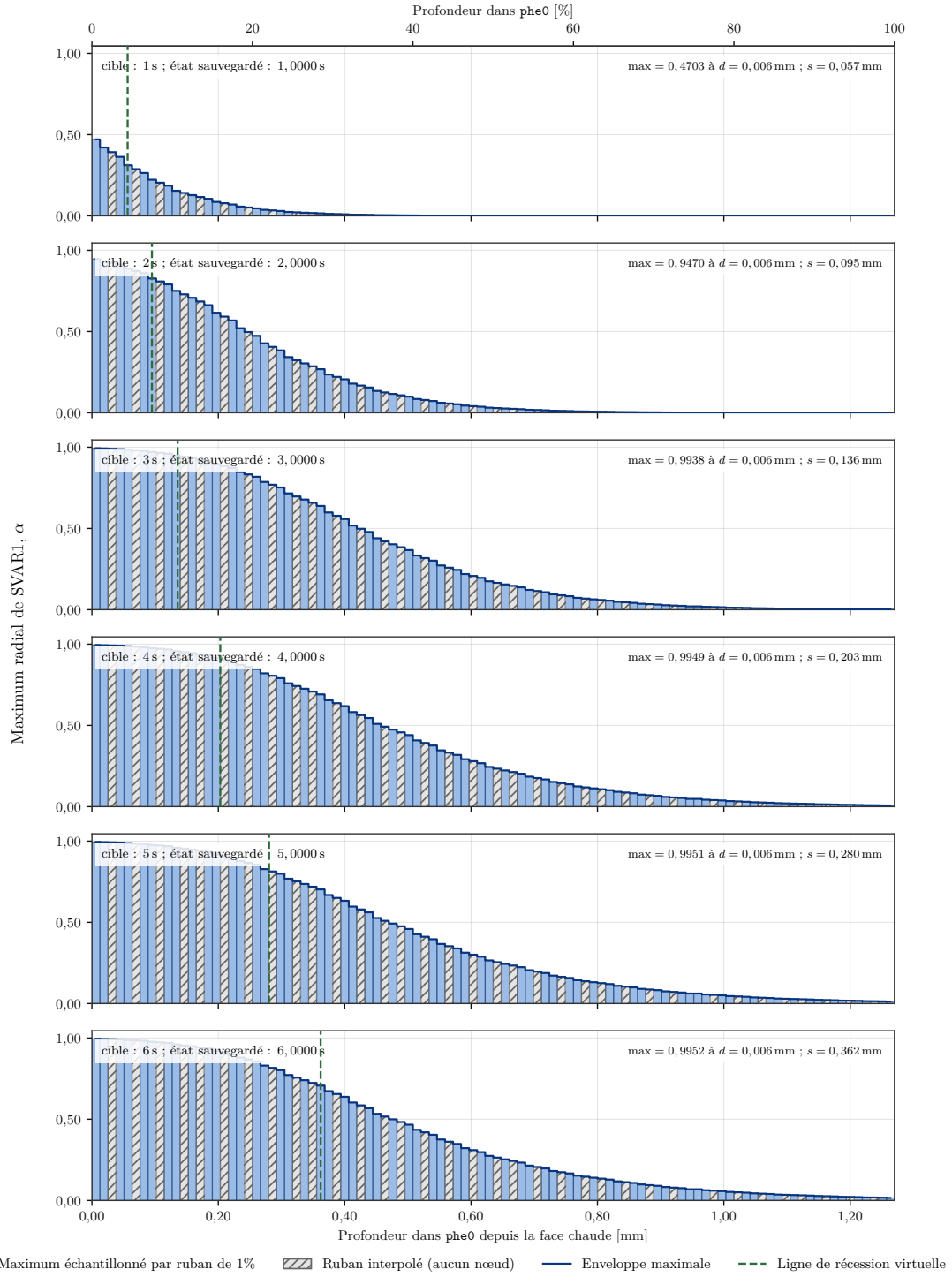
Figure 26. Évolution des profils radiaux de SVAR1 entre 1 et 6 s. La ligne de récession est indiquée dans chaque panneau.
